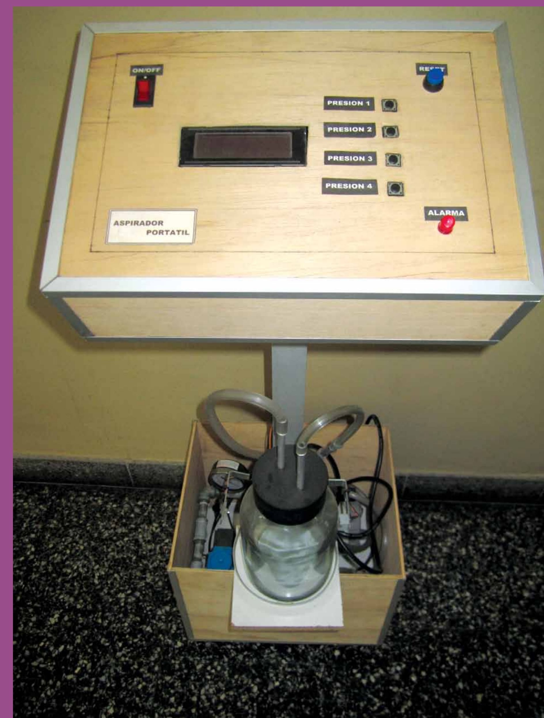
Prototipo de Aspirador de Secreciones
