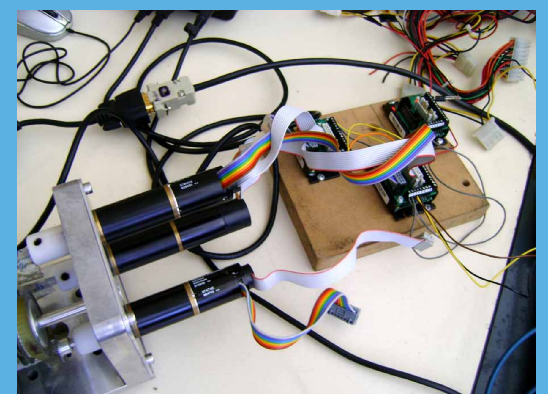
Motor DC e interface de potencia.
